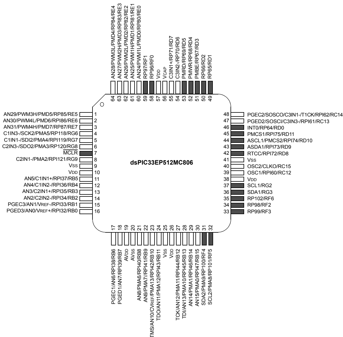
64-Pin TQFP
