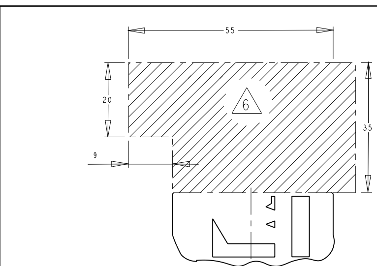
DETAIL G (SCALE: 20:1)
