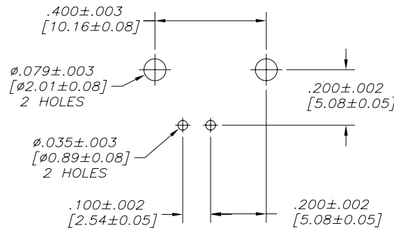
P.C.B. CONFIGURATION
