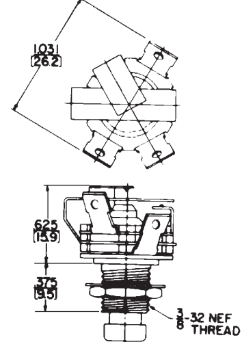
SPDT 1-C
