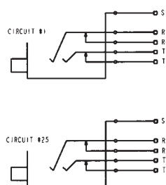
NORMALS OUT TT96EDACNO
