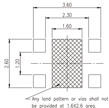
P.C.B. LAYOUT
