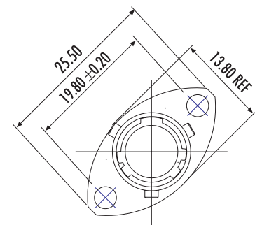
RECEPTACLE - TYPE 0
