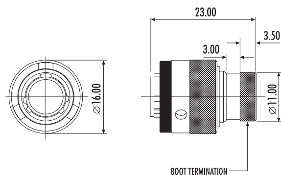
RECEPTACLE - TYPE 0
