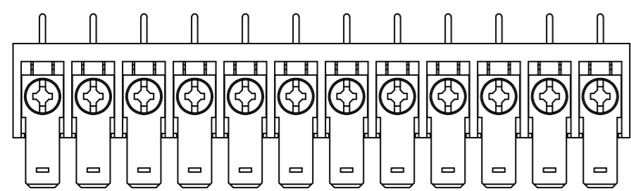
2-796988-9 OBSOLETE .250 TYP
