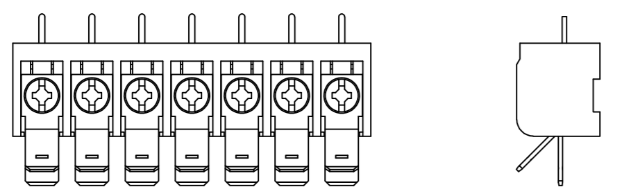
9-1437651-3 .250 TYP
