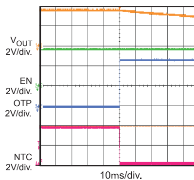
NTC Falling
