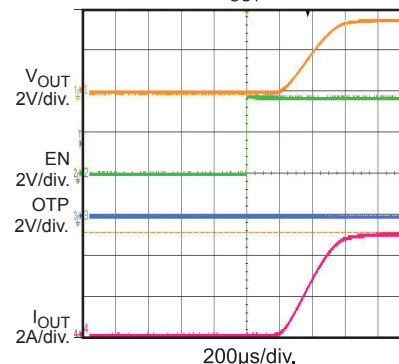
EN Startup
