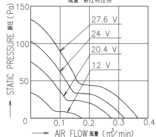
風量-靜壓特性例
