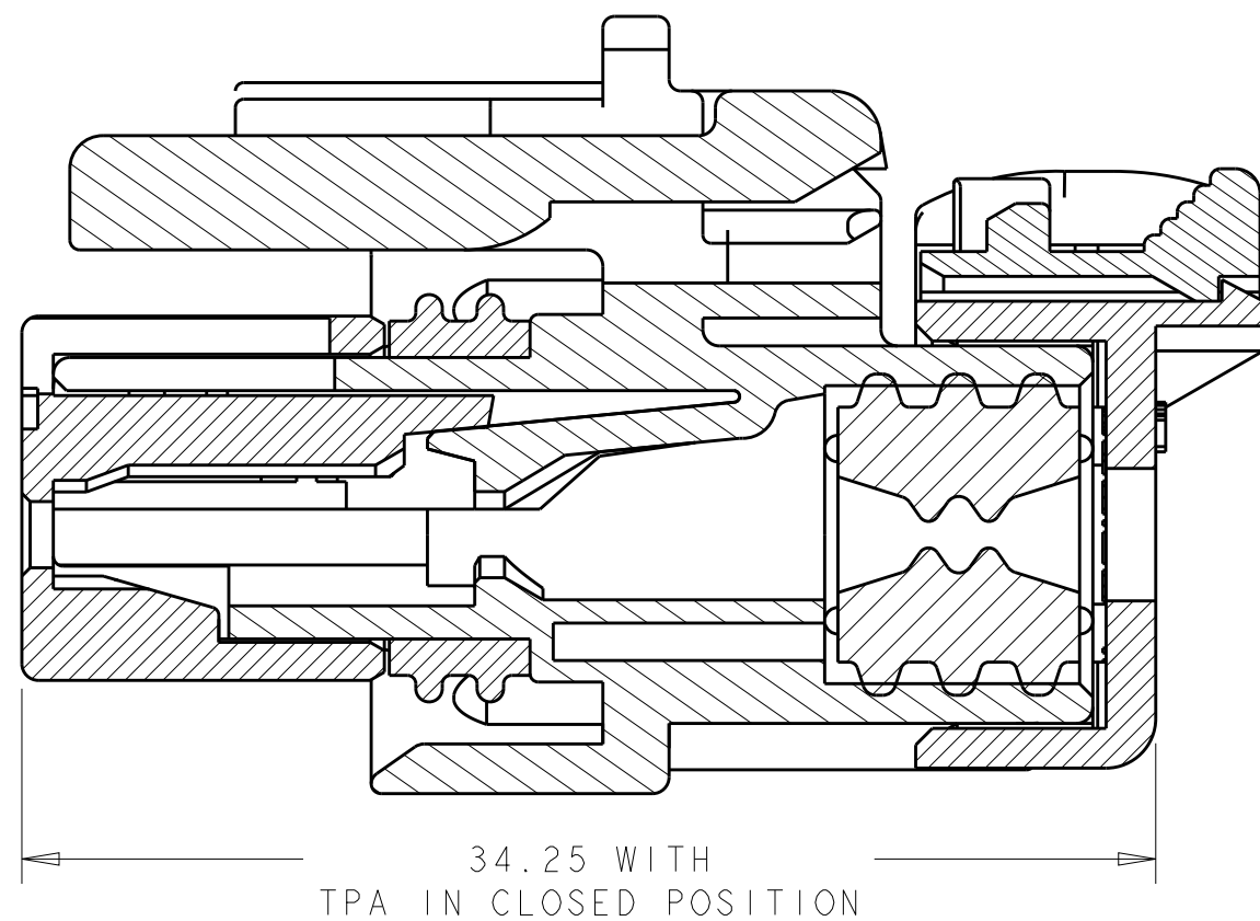
SECTION A-A
