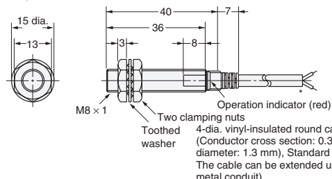
Diagram 9 E2E-X3D□ E2E-X2E□/F□
