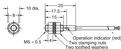
Diagram 4 E2E-X1B□/X1C□
