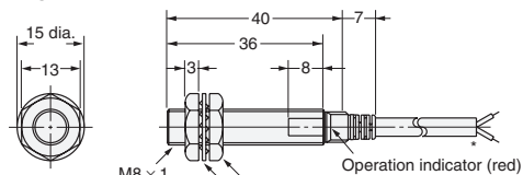
Diagram 7 E2E-X1R5Y□
