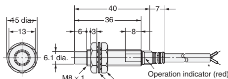
Diagram 8 E2E-X2MY□
