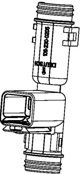
SCALE 1:1 Maßstab
