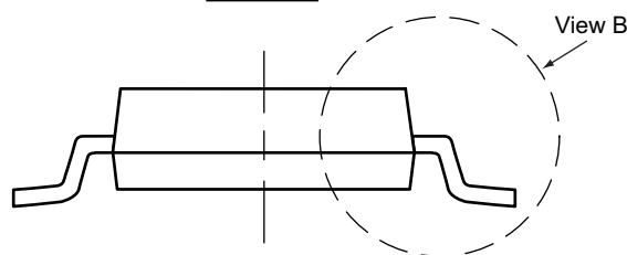
View A-A
