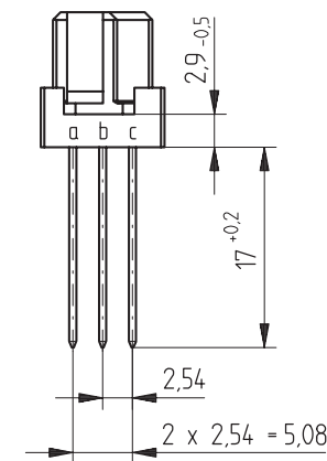
Übergabesteckzone mating transfer zone
