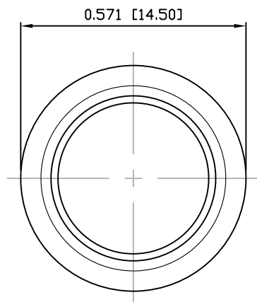
NUT
