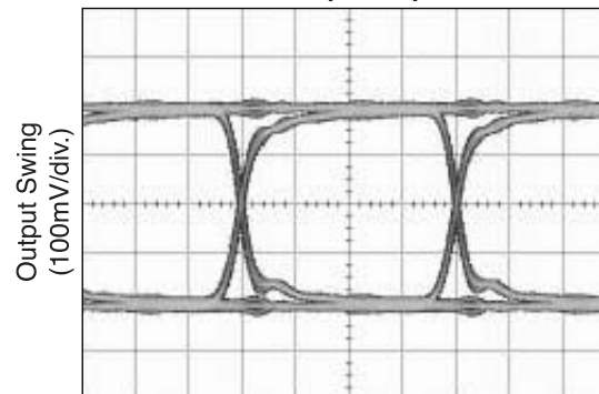
2.5Gbps Output
