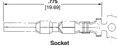
Socket
