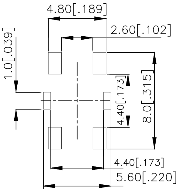
P.C.B LAYOUT
