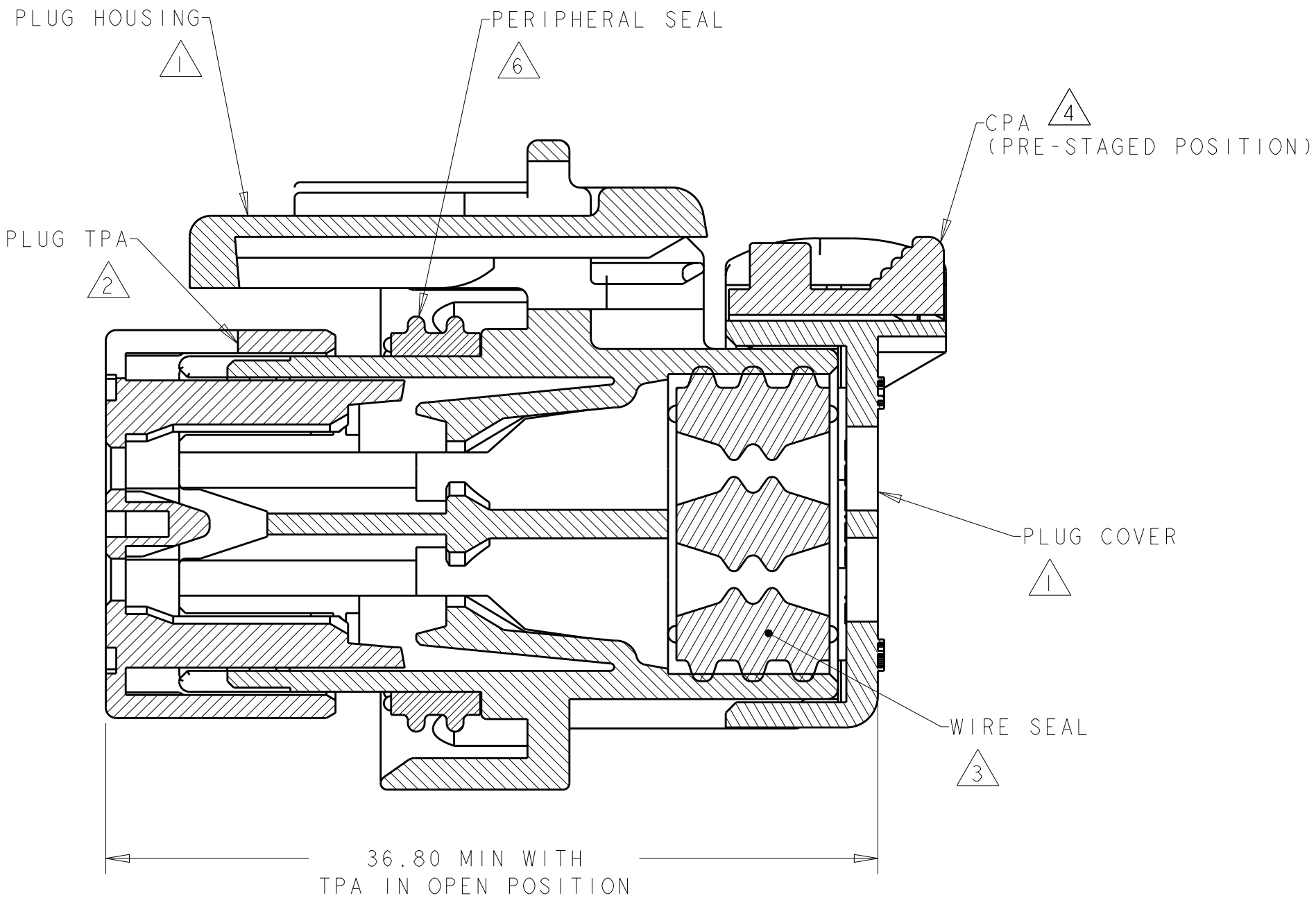
SECTION A-A
