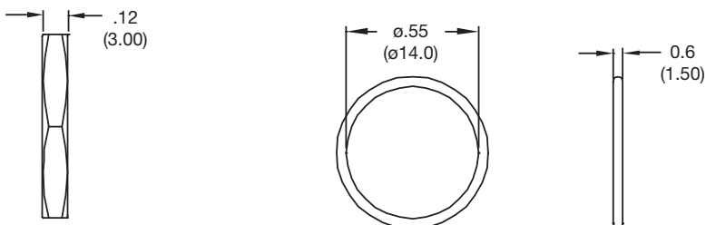
O - RING
