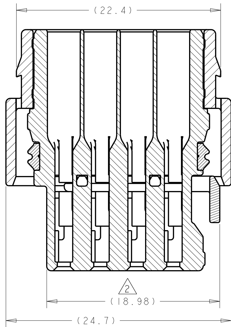
SECTION A-A
