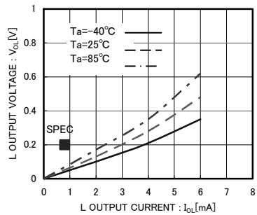
Fig.5 'L' output voltage V_{OL-I_{OL}} ( V_{CC}=1.7V )
