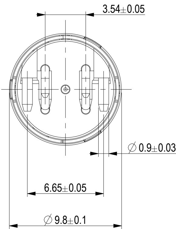
Gemessen über Schirmkontakte Measured over shield contacts
