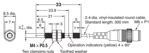
E2E-S04N02-CJ-□□
