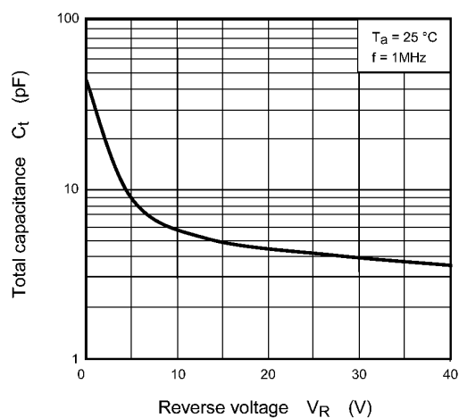
Fig. 9.3 C_t - V_R
