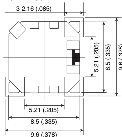
P.C.B. LAYOUT
