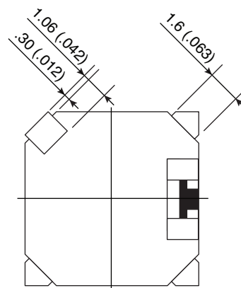
P.C.B. LAYOUT
