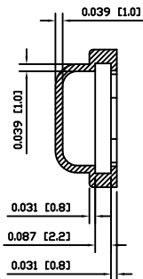
SECTION A-A'
