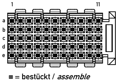
Bestückungsplan / contact layout
