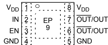
MCP14A1201/MCP14A1202 2 x 3 TDFN*
