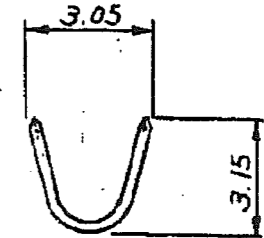
断面 D-D (SECT.)
