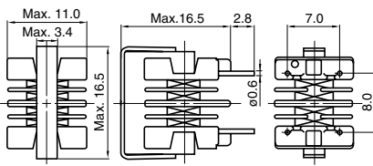
DIMENSIONS (mm) 外形寸法図
