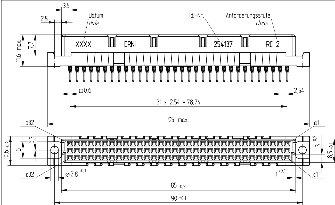
Bestückungsplan / contact layout
