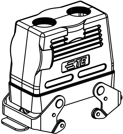
SCALE 1:2
