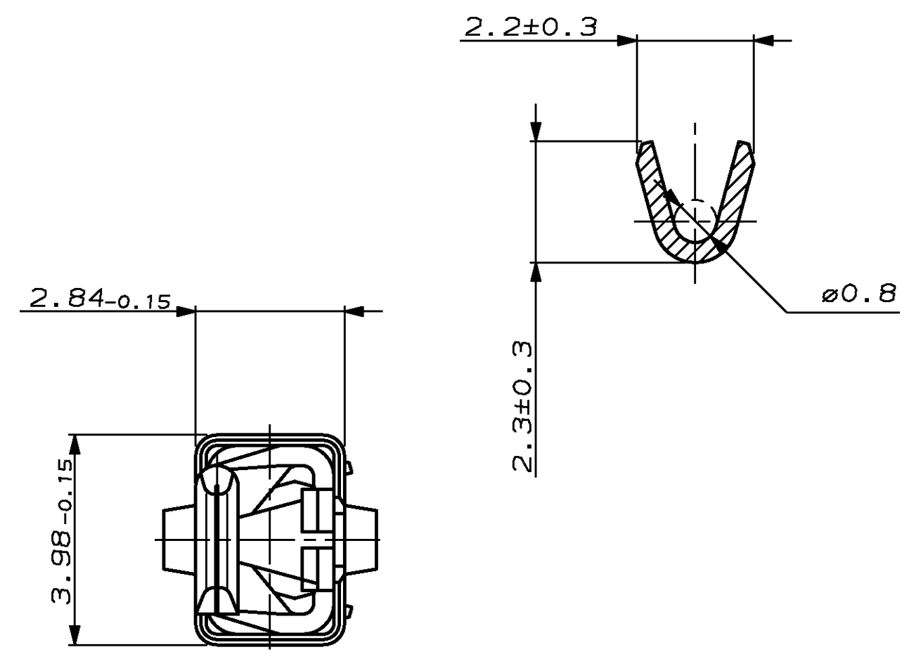
Schnitt A-A
