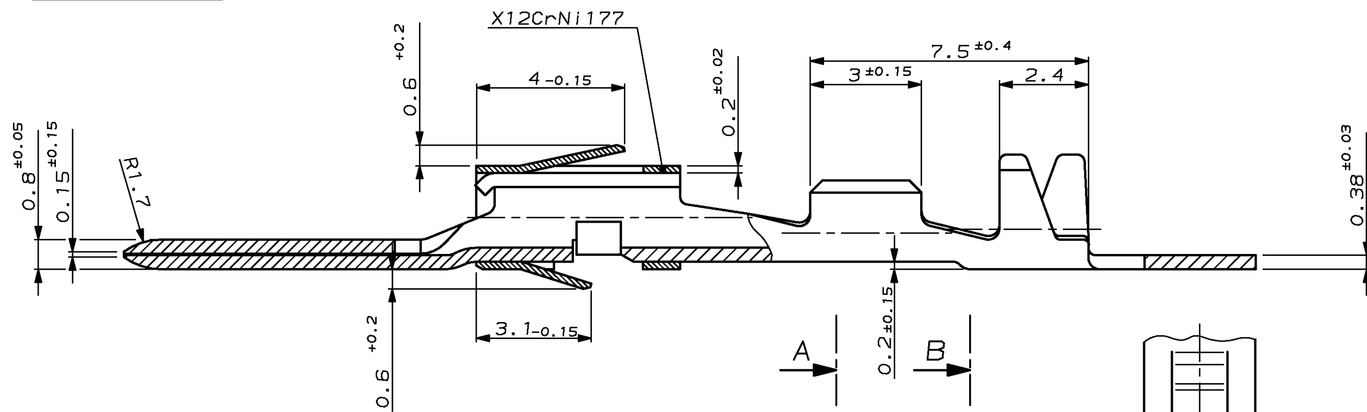
Schnitt B-B
