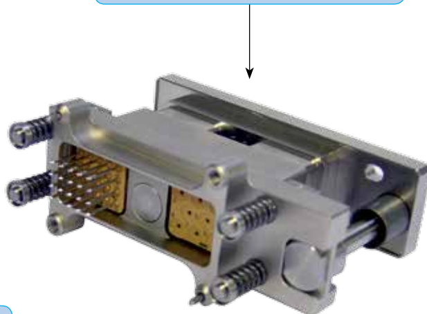
Connecteur rackable métallique 2 modules 2 modules metallic rackable connector
