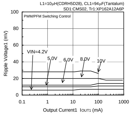
FOSC=500kHz, VOUT1=3.3V
