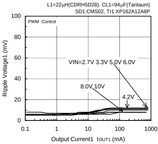
FOSC=300kHz, VOUT1=1.0V
