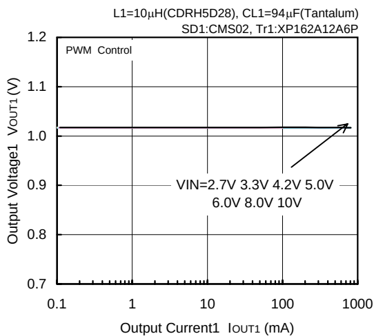
FOSC=500kHz, VOUT1=1.0V
