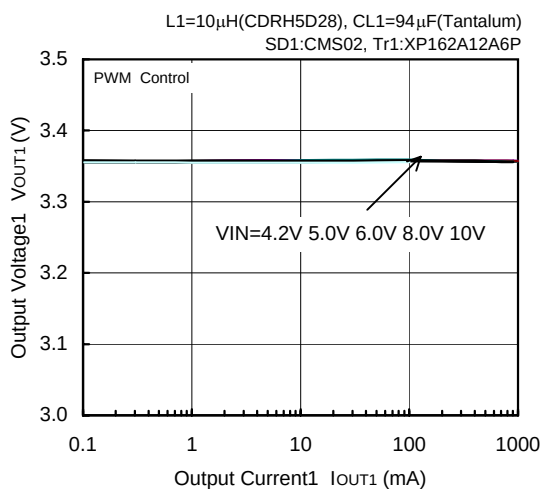
FOSC=500kHz, VOUT1=3.3V
