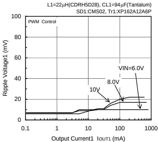
FOSC=300kHz, Vout1=5.0V
