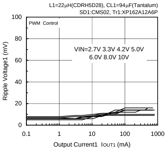
FOSC=300kHz, VOUT1=1.8V
