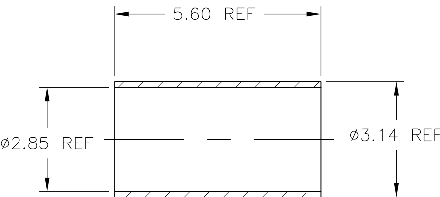
FERRULE
