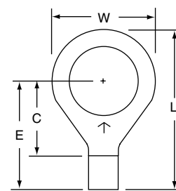
M10-12R
