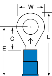
MVU14-14R/S
