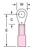
MH18-10R/L
