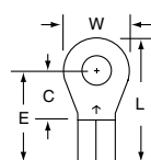
MU10-8R
