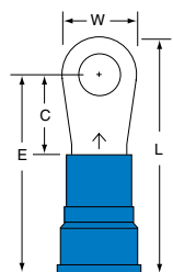
MN6-14R/S
