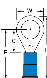
MNG14-516R/S
