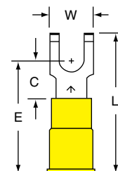
MVU10-10FFBK
