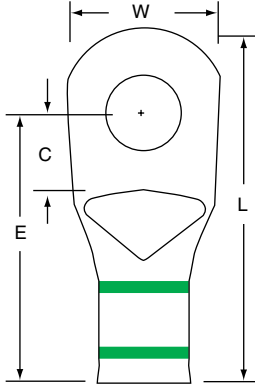
MC1-38RX
