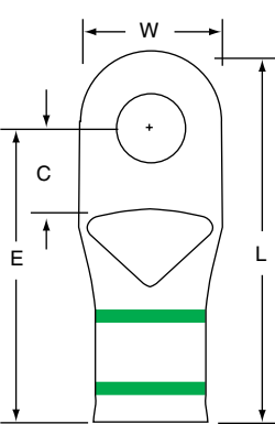
MC1-516RX
