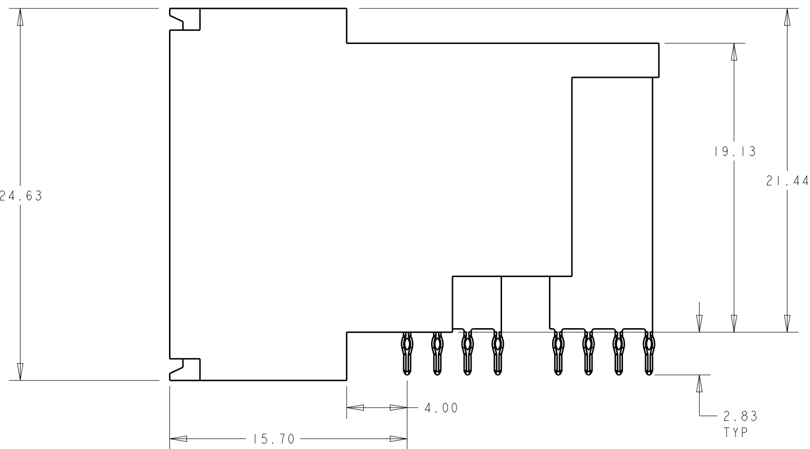
1892711-2 SCALE 3:1
