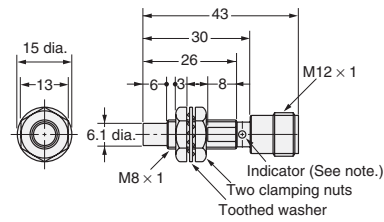
Fig. 18 : E2E-X4MD□-M1(G) E2E-X2ME□-M1/F□-M1
