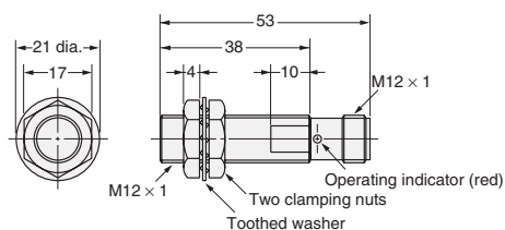
Fig. 23 : E2E-X7D□-M1(G)/E2E-X5E□-M1/F□-M1 E2E-X5Y□-M1
