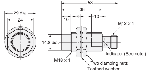
Fig. 24 : E2E-X14MD□-M1(G)/E2E-X10ME□-M1/F□-M1 E2E-X10MY□-M1
