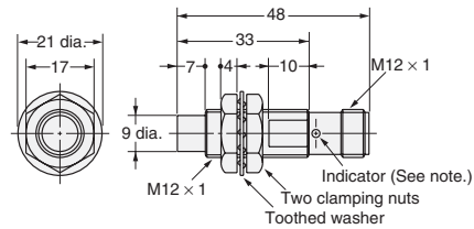
Fig. 20 : E2E-X8MD□-M1(G) E2E-X5ME□-M1/F□-M1
