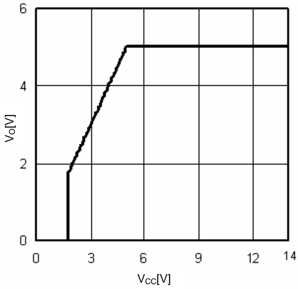
Fig.15 V cc -V o (I o =0mA)
