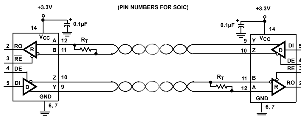
FIGURE 3. ISL3170E, ISL3173E, ISL3176E
