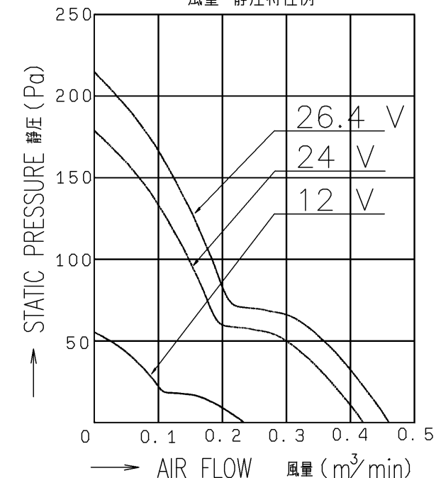
風量-靜壓特性例
