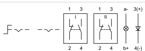
Wiring diagram 24
