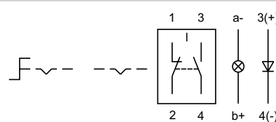
Wiring diagram 20
