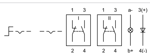
Wiring diagram 24
