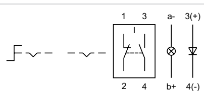
Wiring diagram 20
