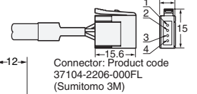
Diagram 15 E2E-X14MD□/E2E-X10ME□/F□ E2E-X10MY□
